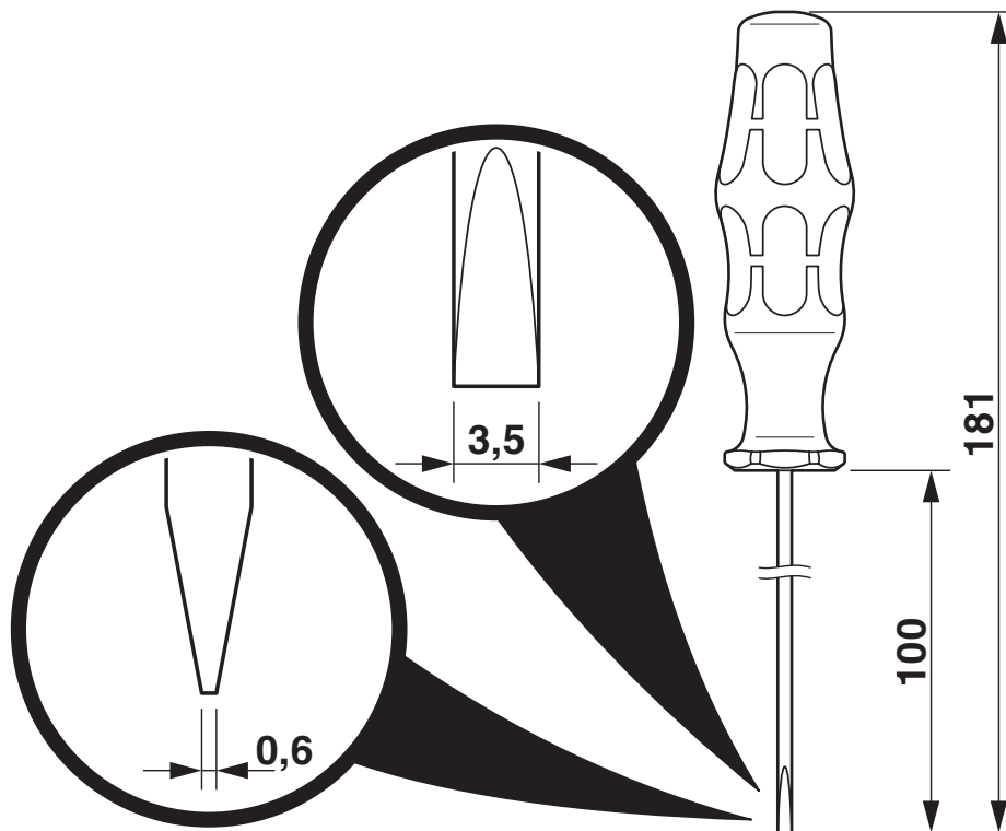
尺寸图
