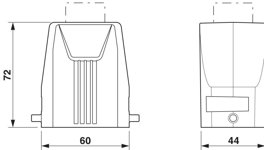
尺寸图
