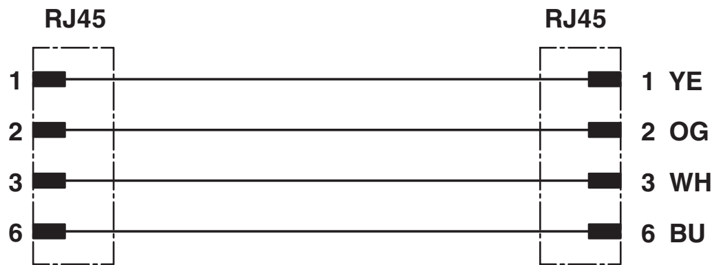
电路图
