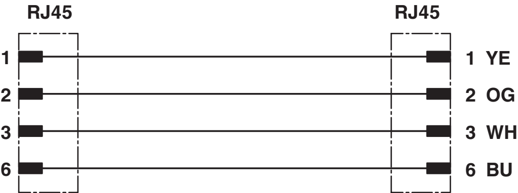
电路图
