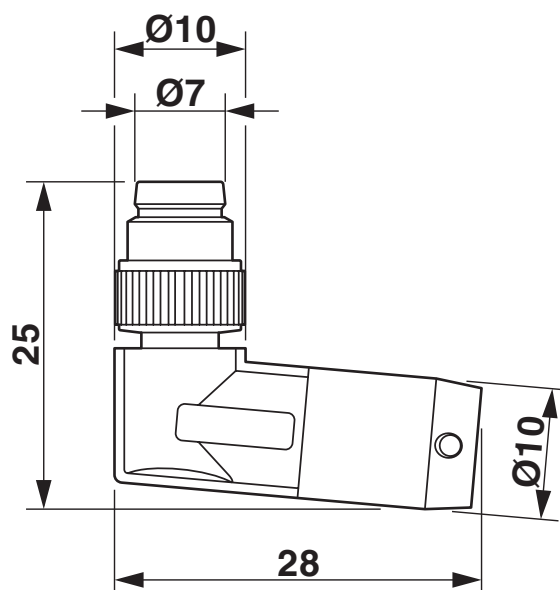
尺寸图
