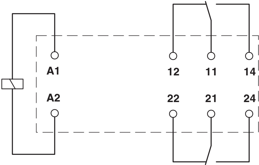
电路图
