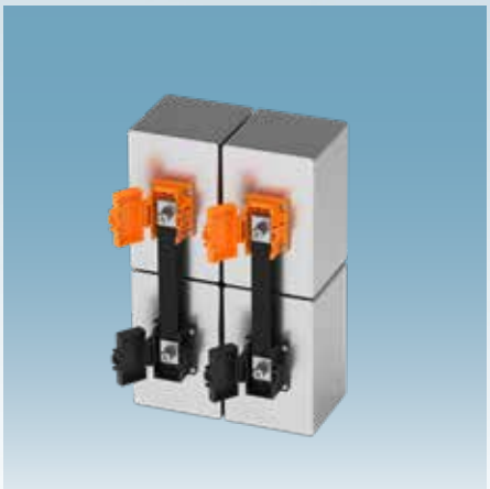
储能电池模块系统穿墙式连接器 可实现安全、经济且高效地安装储能模块系统。
