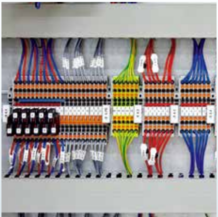
直插自锁式接线端子 无需工具即可轻松完成导线连接。采用特殊的触点弹簧，导线轻松插入省力 50%，连接牢固可靠。可选正面和侧面接线的不同产品系列。
