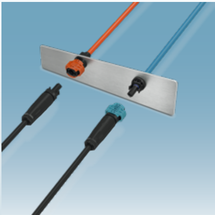
SUNCLIX 储能连接器 正负极颜色及键位机械防错插设计，弹簧接线，布线方便。
