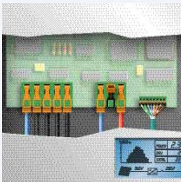
用于逆变器 PCB 板的连接技术
