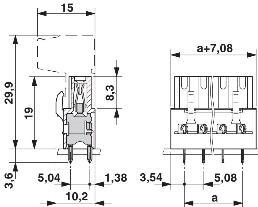
尺寸图
