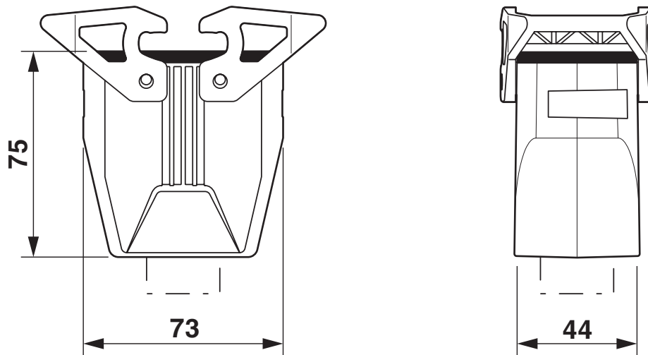
尺寸图
