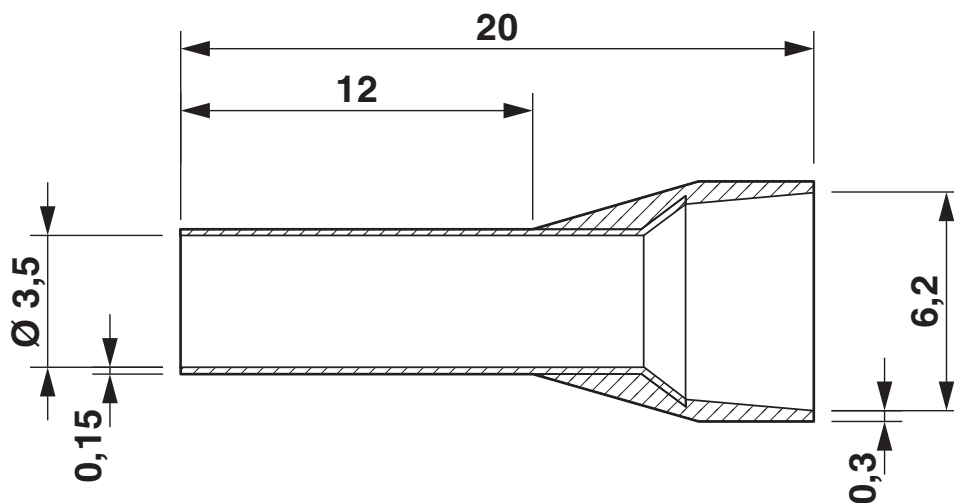
尺寸图
