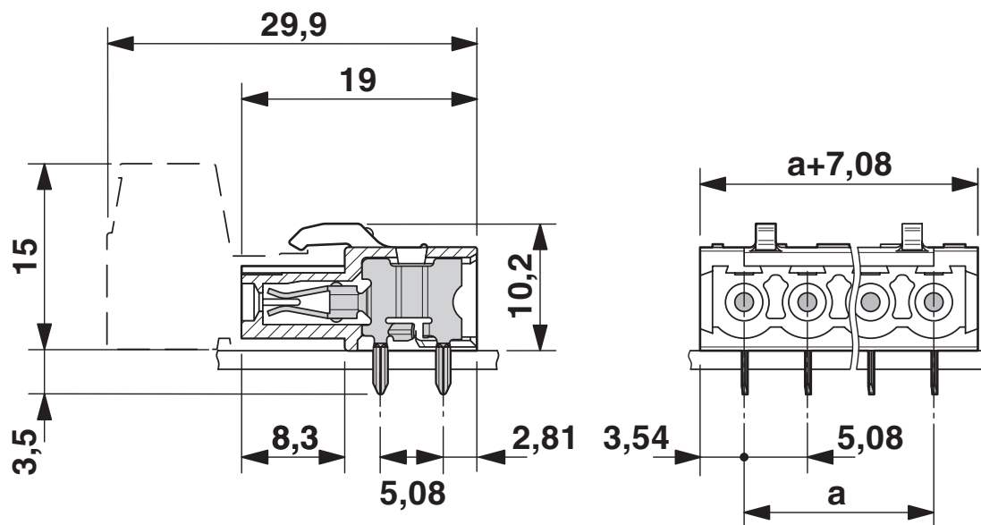
尺寸图
