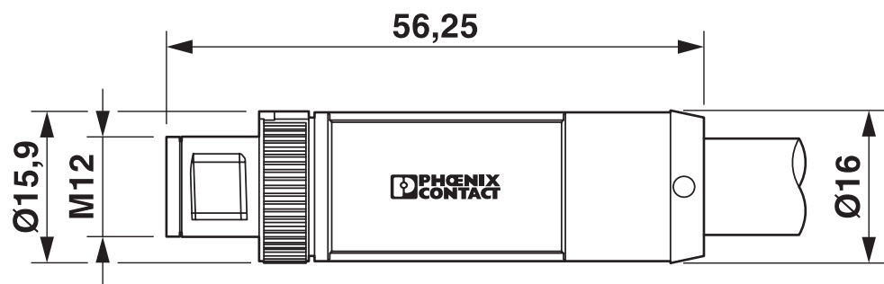
尺寸图
