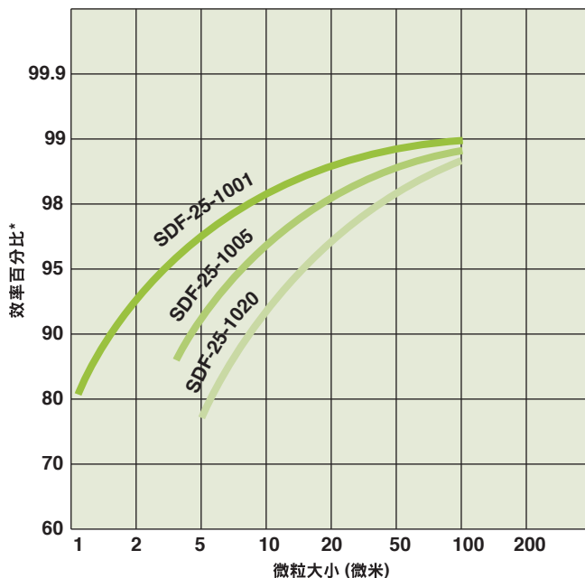
直徑 2.5 吋 X 長度 9 7/8 吋
