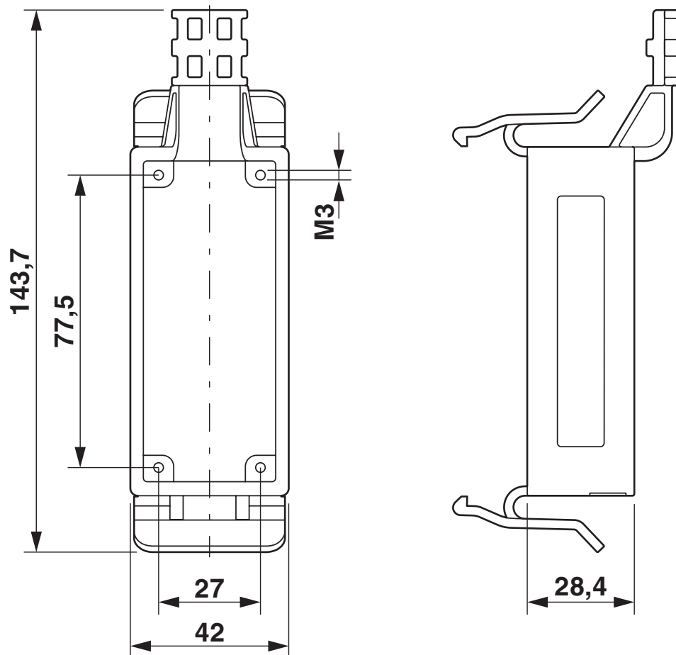
尺寸图
