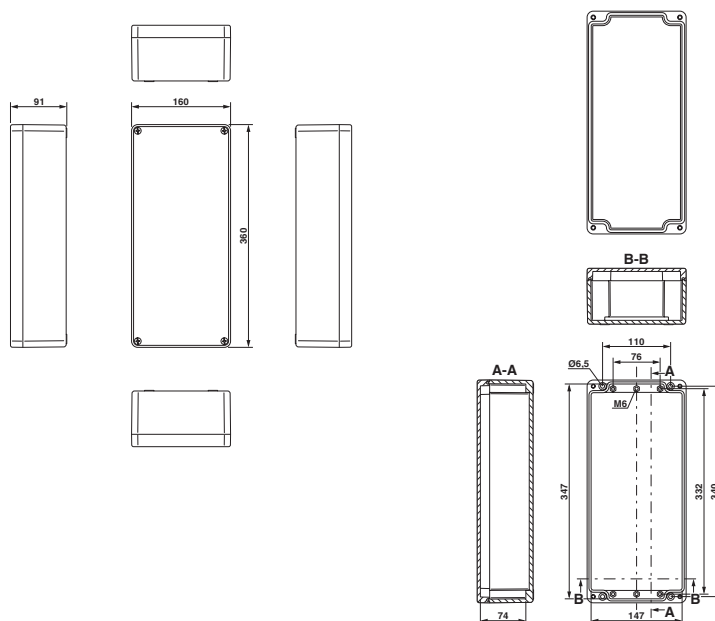
尺寸图
