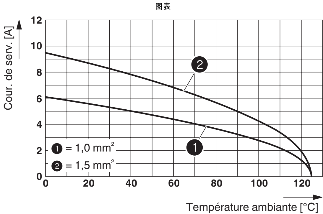
衰减曲线图（HC-B 24外壳可容纳3个模块）
