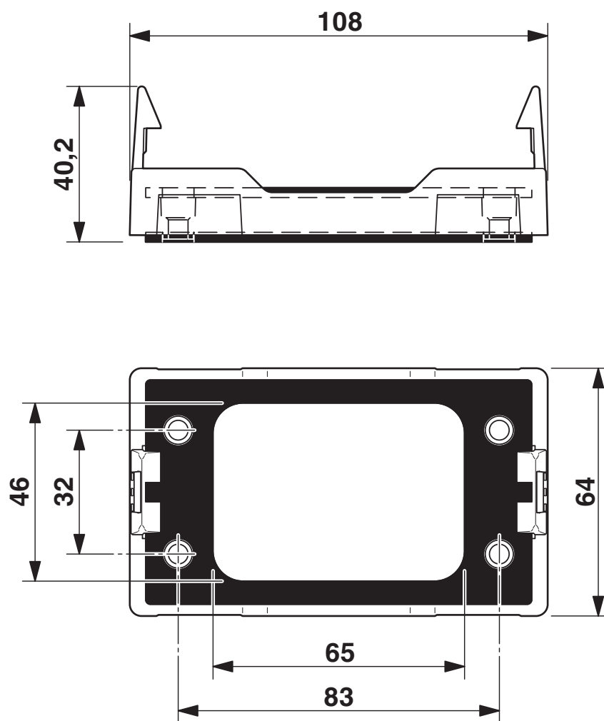
尺寸图
