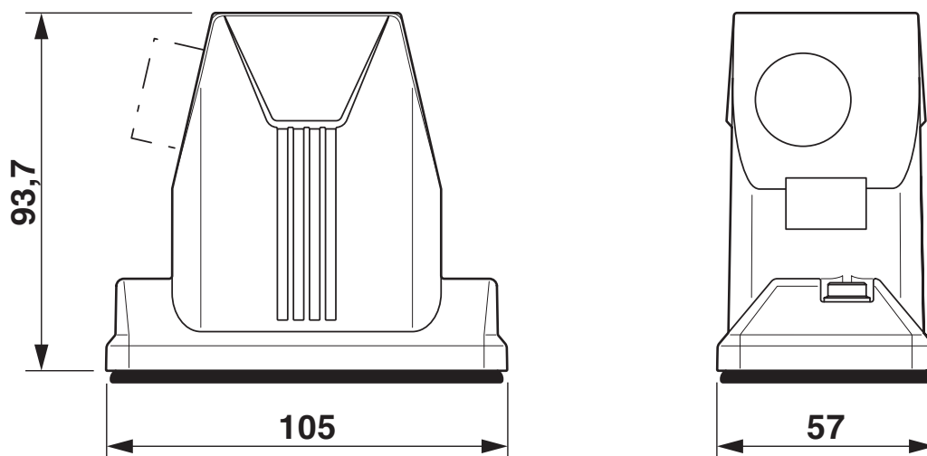
尺寸图
