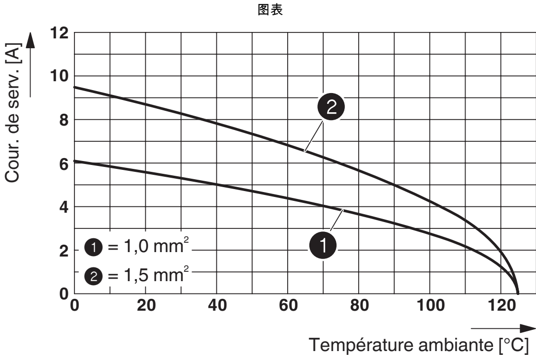
衰减曲线图（HC-B 24外壳可容纳6个模块）
