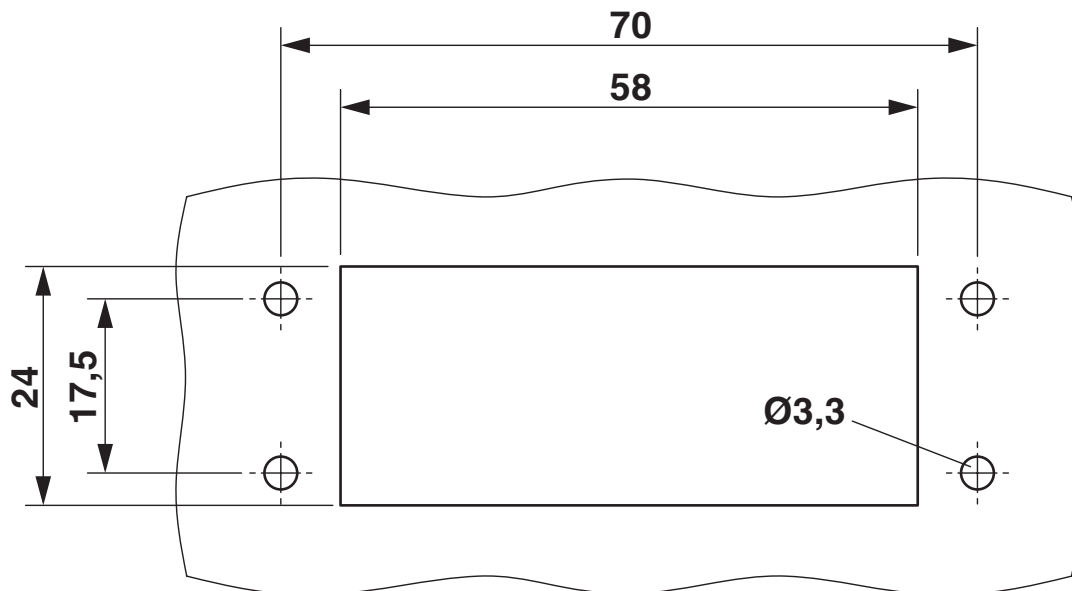
尺寸图
