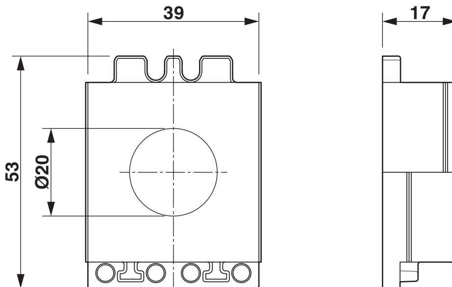
尺寸图
