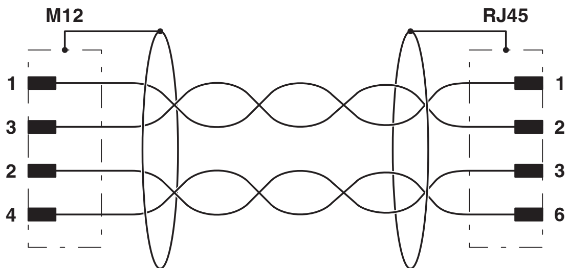
电路图
