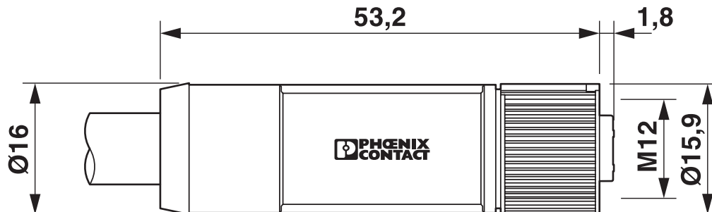
尺寸图
